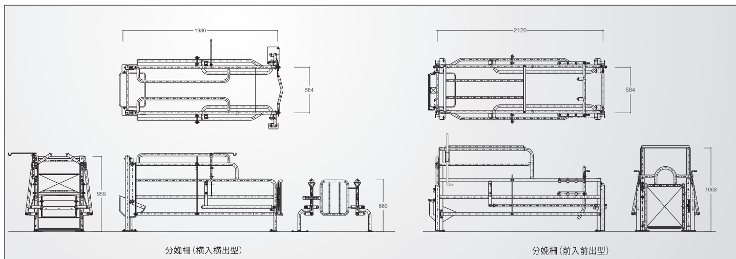
横入横出型（縦配置）
